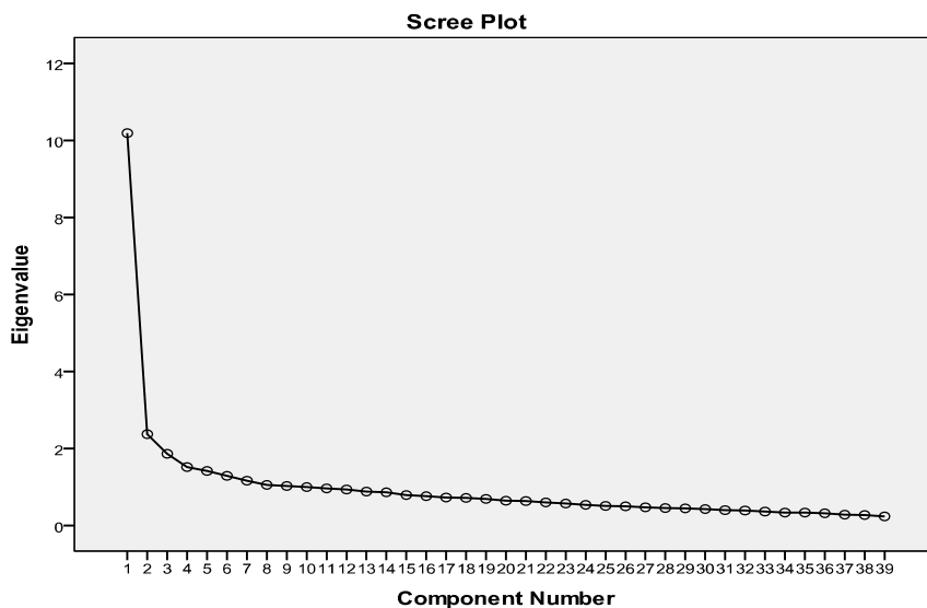
شکل ۱- نمودار اسکری.
